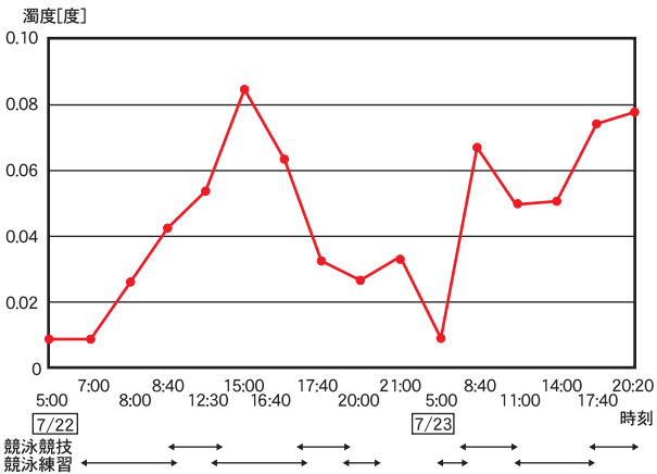
図 5 濁度変化
