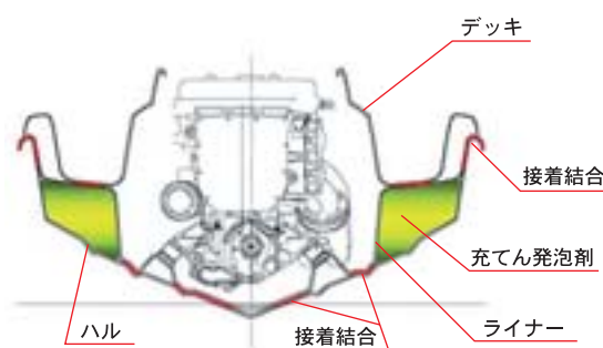
図3 船体構造図
