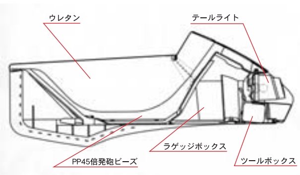
図 9 シート断面図
