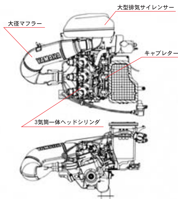
図 3 SXV70 エンジン
