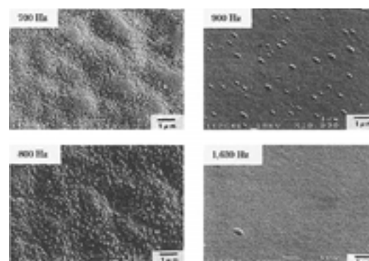
図3 周波数の変化に応じた表面形態
