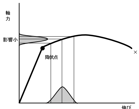
図6 ボルトの塑性域締付け
