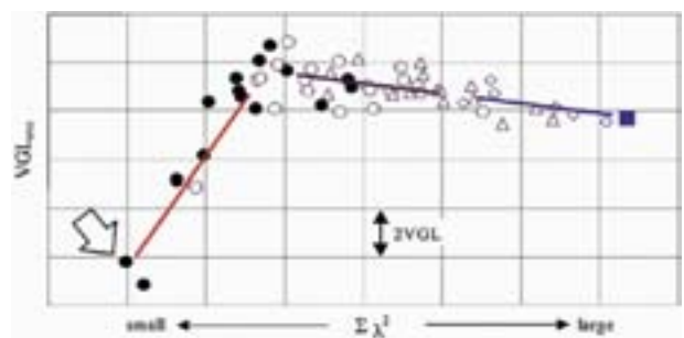
図4 FEモデルによる振動予測結果
