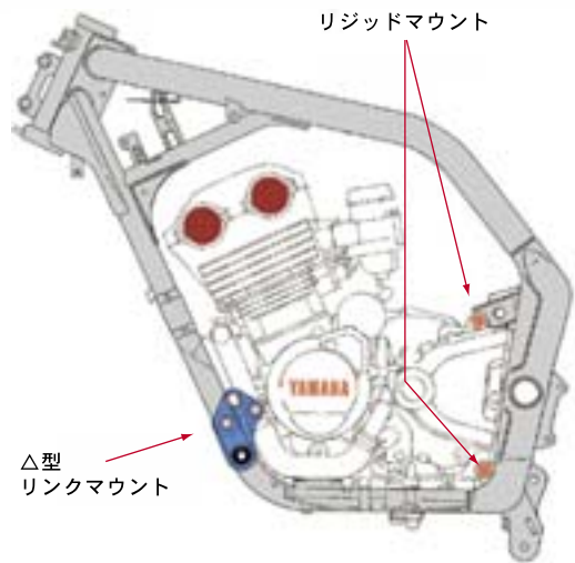
図5 △型リンクマウント
