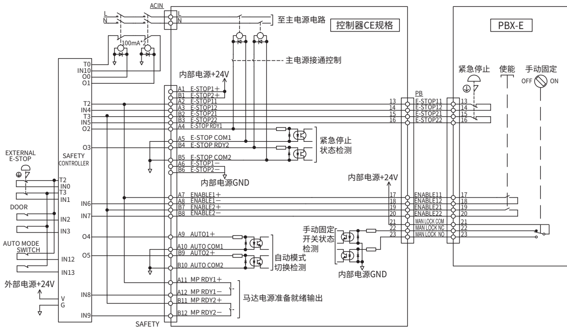
● CE规格控制器与PBX-E的连接示例
