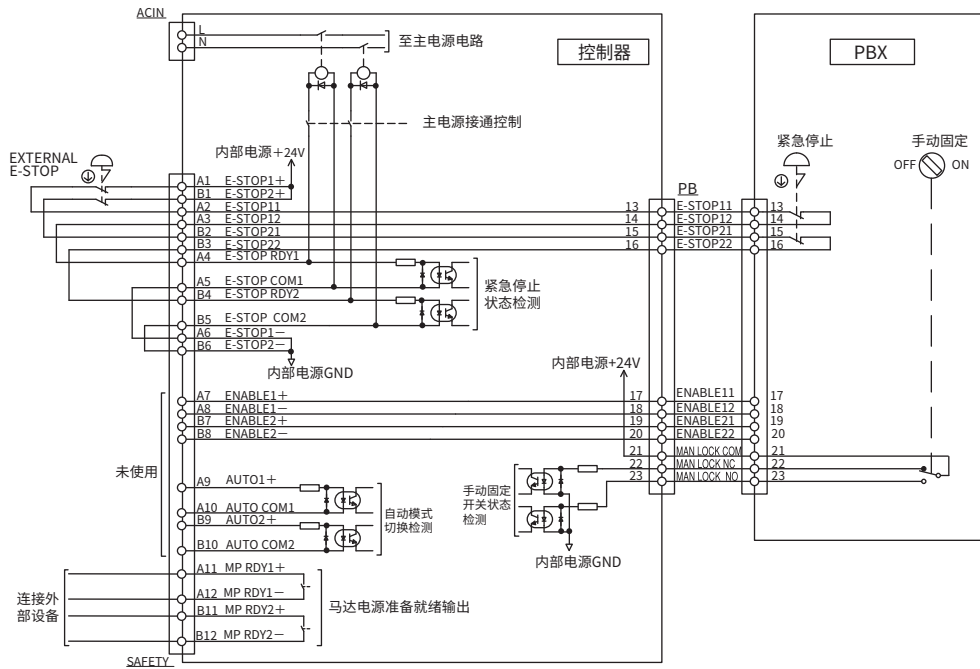
● 普通规格控制器与PBX的连接示例
