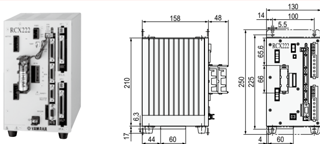
RCX222 Dimensions
