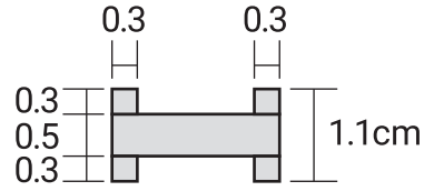
C 断面図
