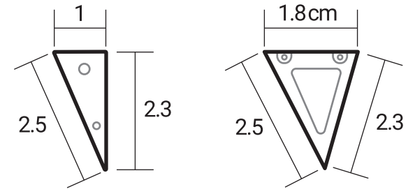
フェンダーステー FP-14
