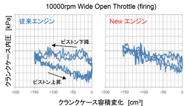
図4 クランクケース内P-V線図
